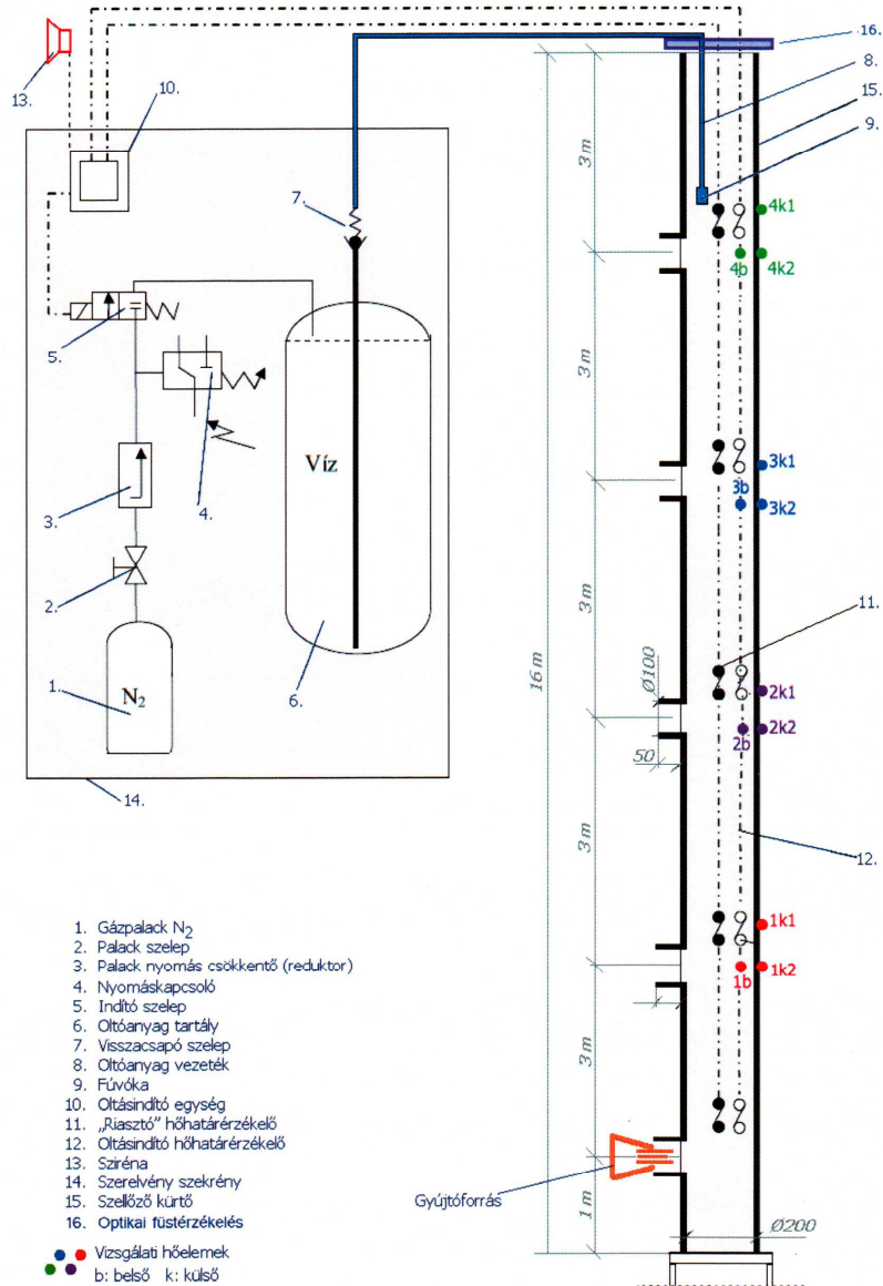
1. ábra Vizsgálati berendezés (1. és 2. vizsgálatnál) Tűjelző, füst-, hő-, és tüztovaterjedésgátló berendezés Típus: VSZ120-200 RT
