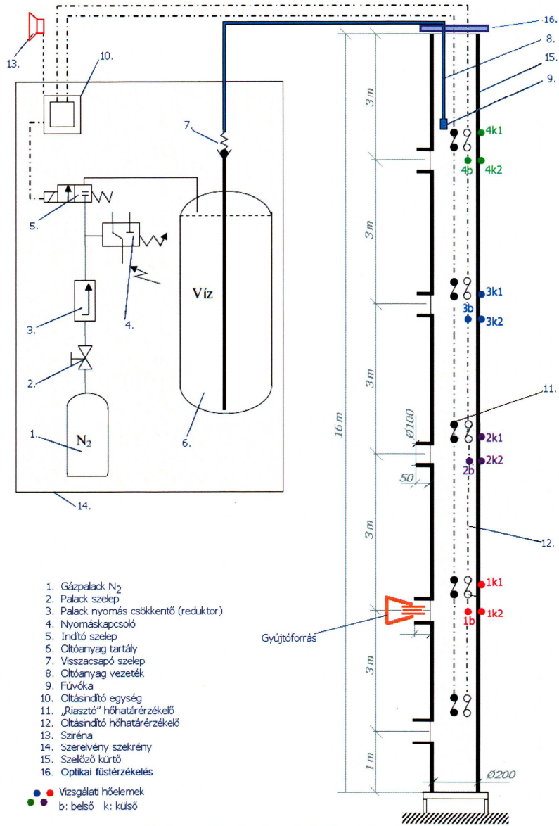
2. ábra Vizsgálati berendezés (3. vizsgálatnál) Tűzjelző, füst-, hő-, és tűzovaterjedésgátló berendezés Típus: VSZ120-200 RT
